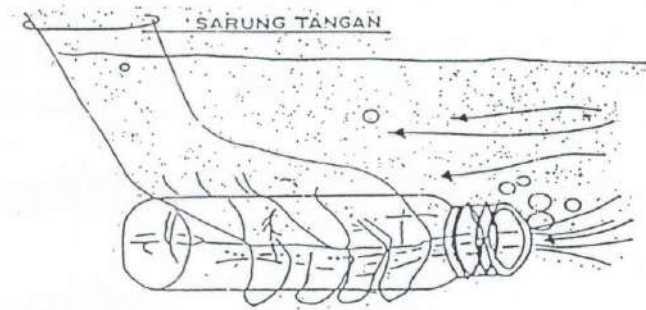
Gambar 8. 3. Contoh alat pengambil air botol biasa secara langsung
