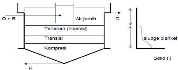
Gambar 7. 9. Pengendapan final clarifier pada proses lumpur aktif
