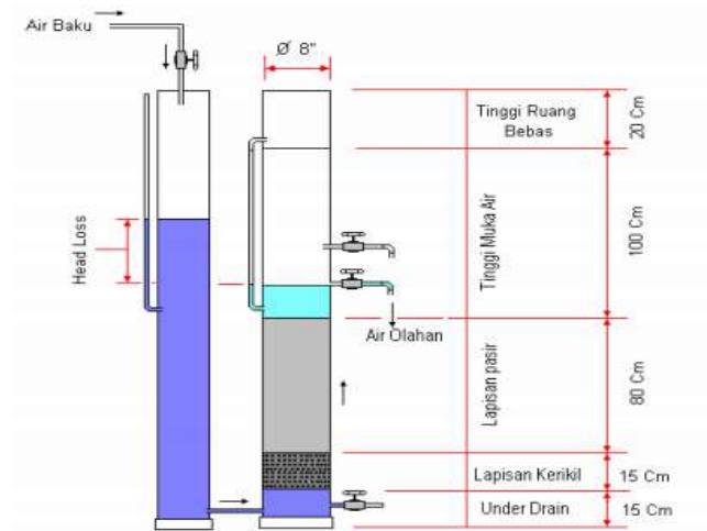
Gambar 7. 7. Saringan pasir dengan mekanisme tekanan ( up low )
