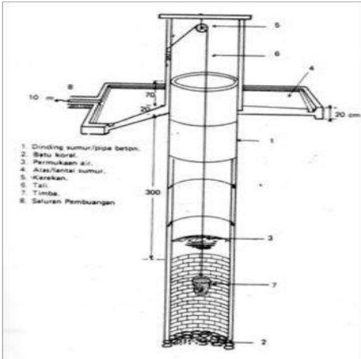
Gambar 4. 2. Penampang Vertikal Sumur Gal
