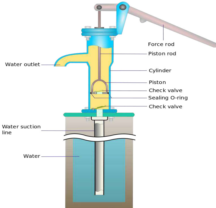
Gambar 4. 4. Sumur pompa tangan dangkal
