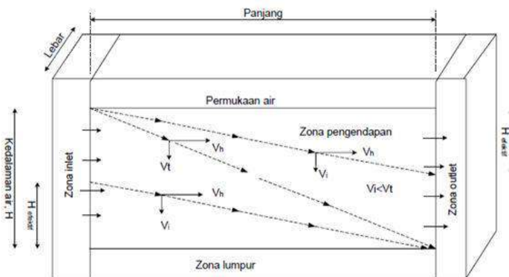
Gambar 7. 11. Bagian dari bak sedimentasi
