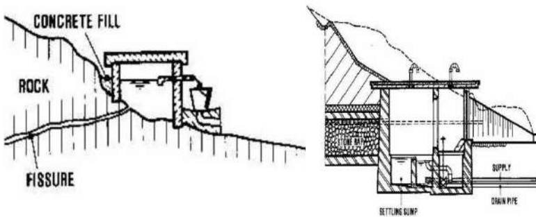
Gambar 4. 7. Bak perlindungan mata air
