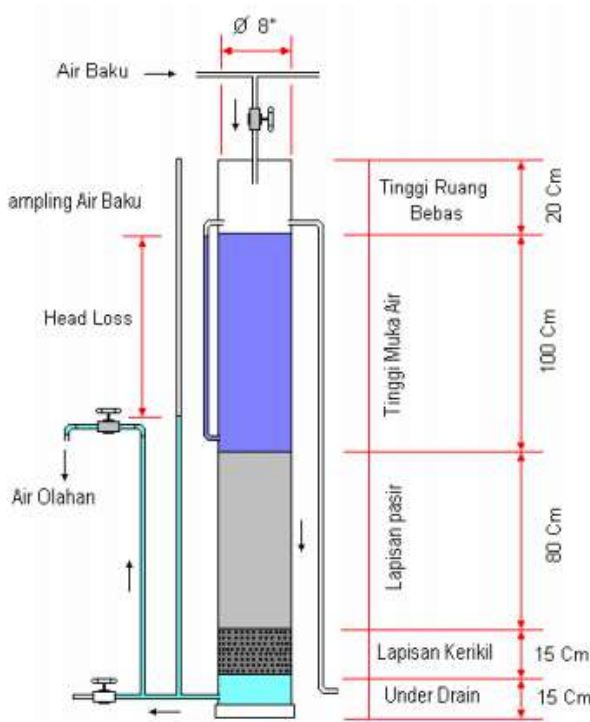
Gambar 7. 6. Saringan pasir dengan mekanisme gravitasi ( Down Flow )
