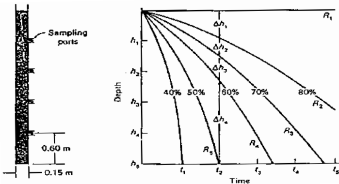
Gambar 7. 8. Kolom pengendapan dan kurva pengendapan partikel flok
