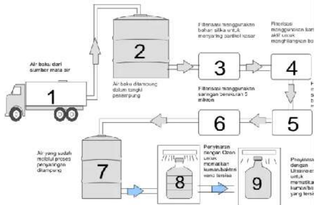
Gambar 7. 16. Alur pengolahan air pada depot
