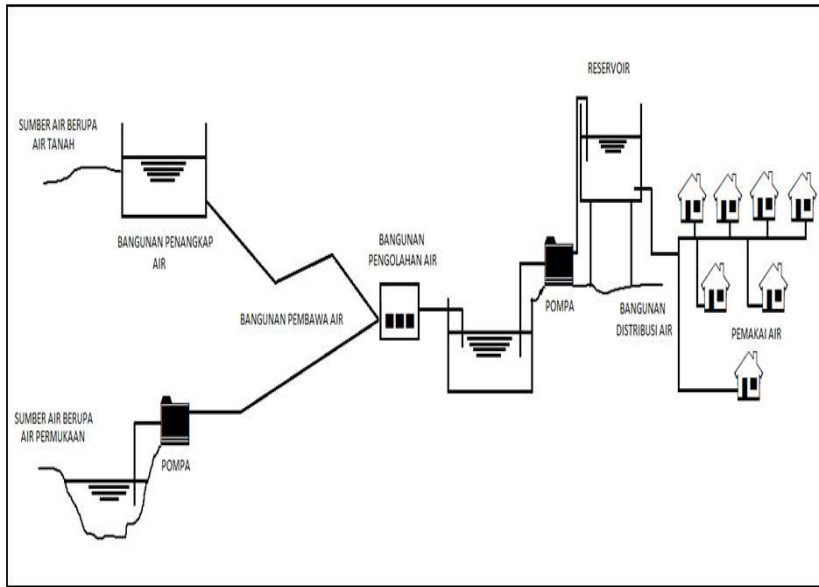
Gambar 4. 10. Sarana air bersih perpipaan
