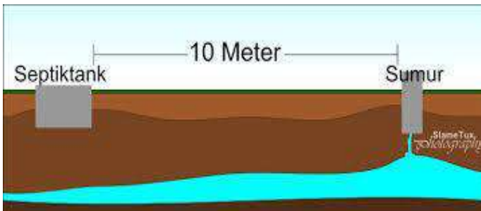
Gambar 5. 2. Jarak sumur gali dengan septic tank
