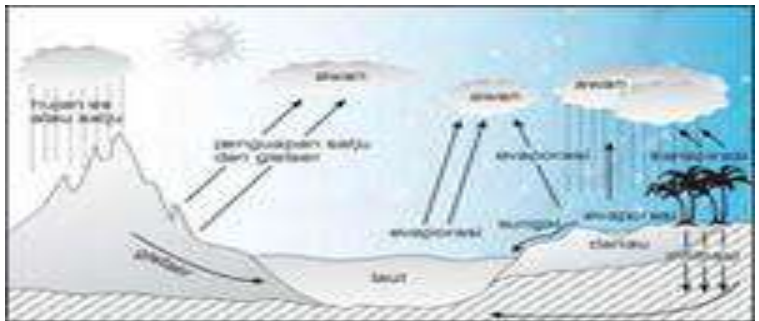
Gambar 1. 5. Siklus air panjang
