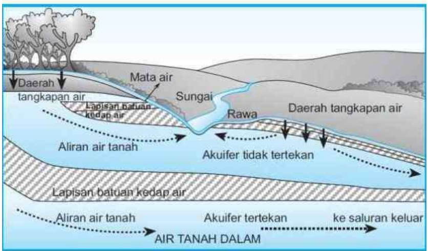
Gambar 2. 4. Proses terbentuknya air tanah
