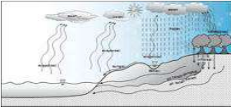
Gambar 1. 4. Siklus air sedang
