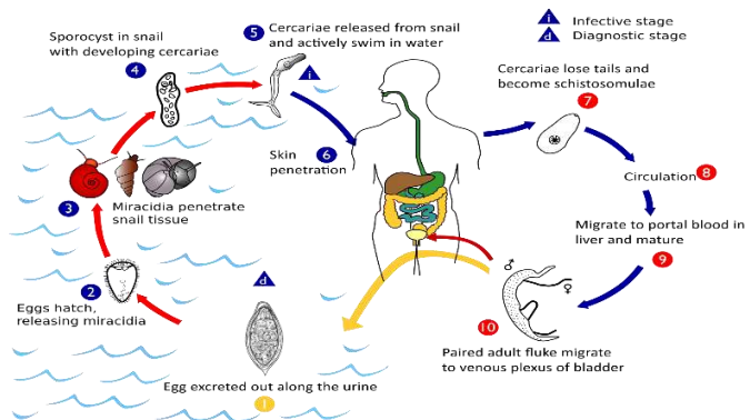
Gambar 5. 4. Mekanisme penularan penyakit skistosomiasis
