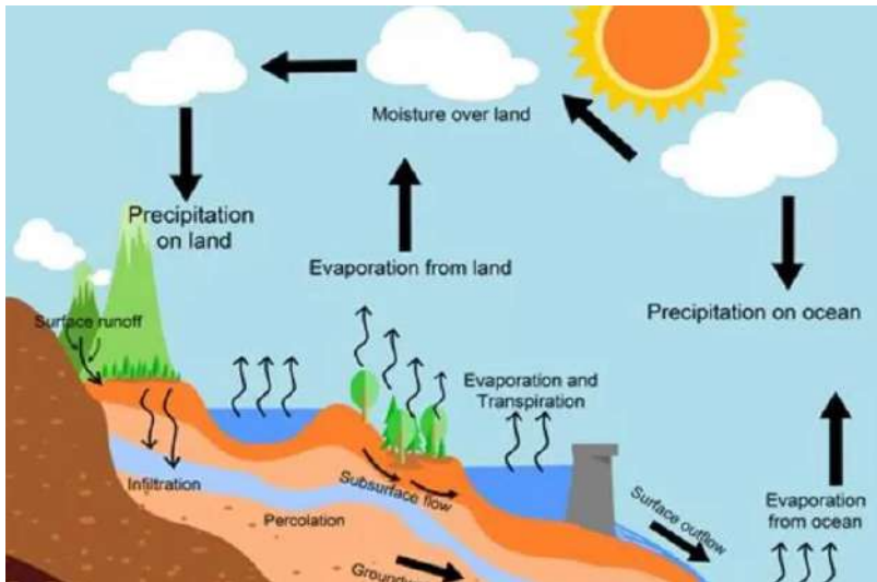
Gambar 1. 2. Siklus air di bumi
