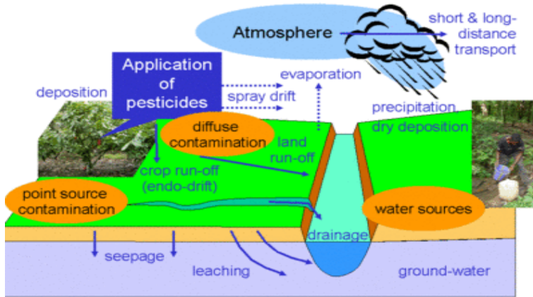
Gambar 3. 6. Mekanisme pencemaran air oleh penggunaan pestisida
