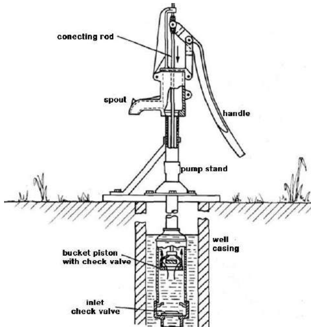
Gambar 4. 5. Sumur pompa tangan dalam
