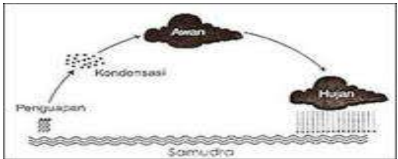
Gambar 1. 3. Siklus air pendek
