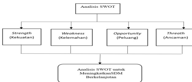
Gambar 11.1 Kerangka Konseptual
