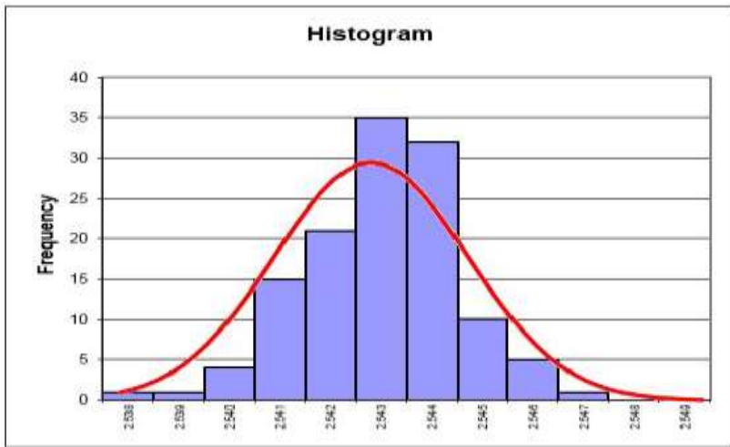
Gambar 9.5. Contoh Histogram
