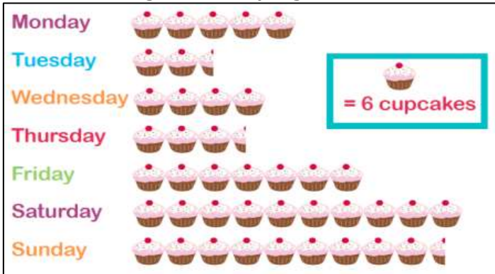
Gambar 9.13. Contoh Pictogram
