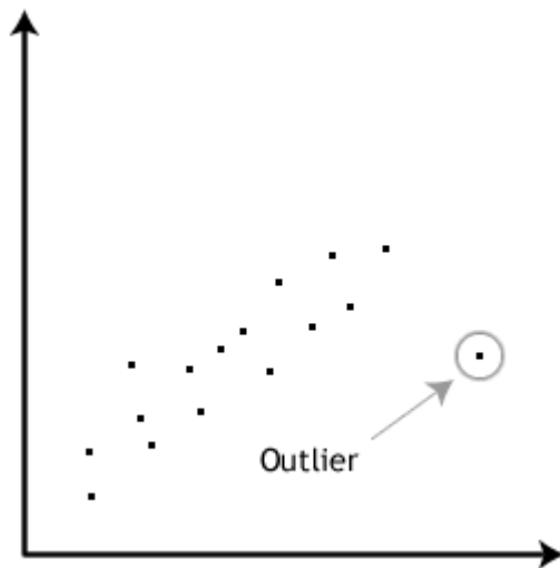
Gambar 11.6. Outlier
