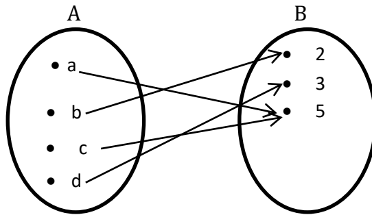
Gambar 4. Fungsi Surjektif
