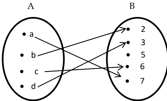
Gambar 3. Fungsi Injektif
