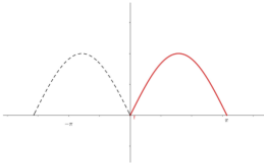
Gambar 4.9 Grafik f(x) = \sin x
