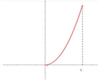
Gambar 4.4 Fungsi f pada Domain [0,L]
