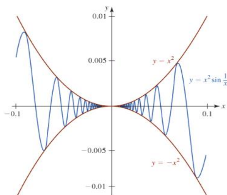
Gambar 7.5 Grafik fungsi f, g dan h
