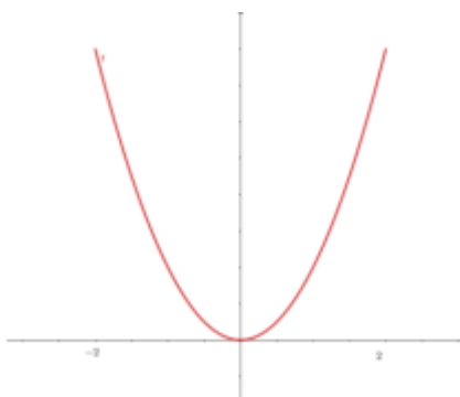
Gambar 4.7 Grafik Fungsi f(x) = x^2
