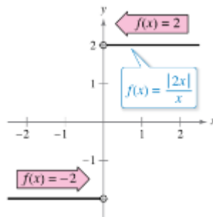
Gambar 7.3 grafik fungsi f(x) = \frac{|2x|}{x}
