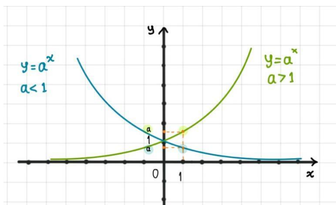
Gambar 5.2 Grafik Fungsi y = a^x , dengan a > 1 dan a < 1
