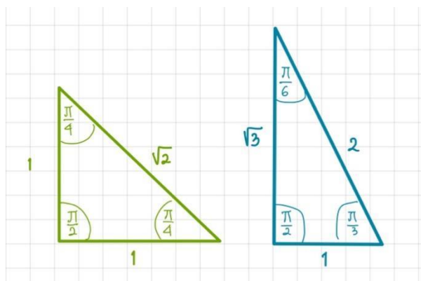
Gambar 5.6 Sudut Radian dan Panjang Sisi Segitiga Siku-siku
