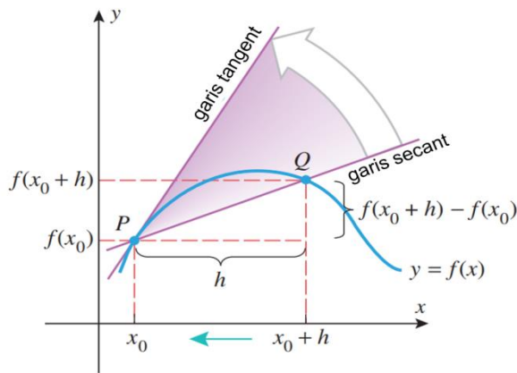
Gambar 9.3 Gradien Garis Tangent sebagai Limit dari Garis Secant
