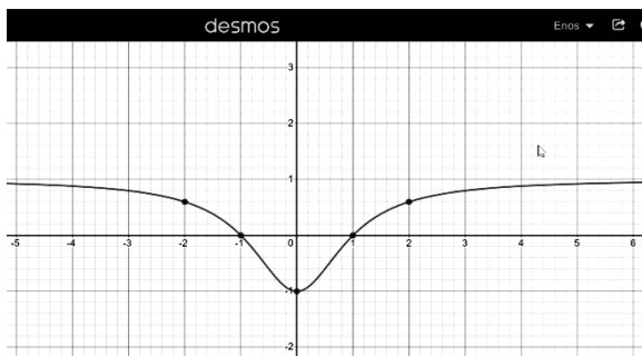
Gambar 6.13 Limit di tak-hingga
