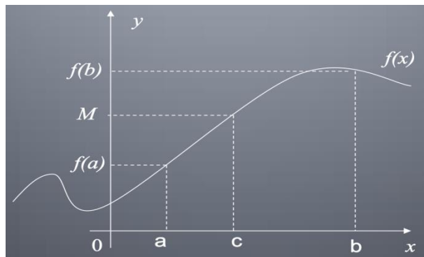
Gambar 8.6 Grafik fungsi Teorema Nilai Antara
