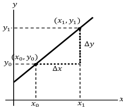
Gambar 9.1 Garis yang Melalui Titik (x_1, y_1) dan (x_2, y_2)
