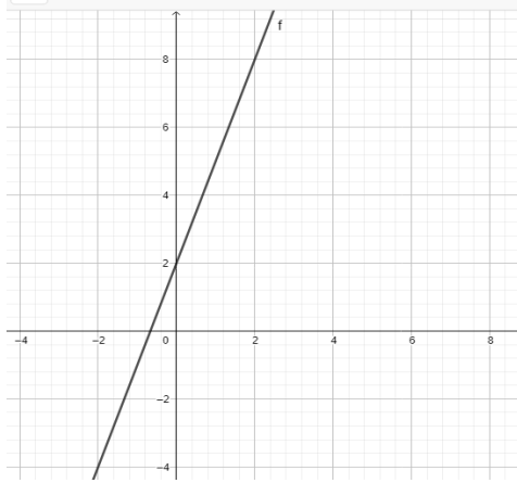
Gambar 4.1 Grafik Fungsi Linier
