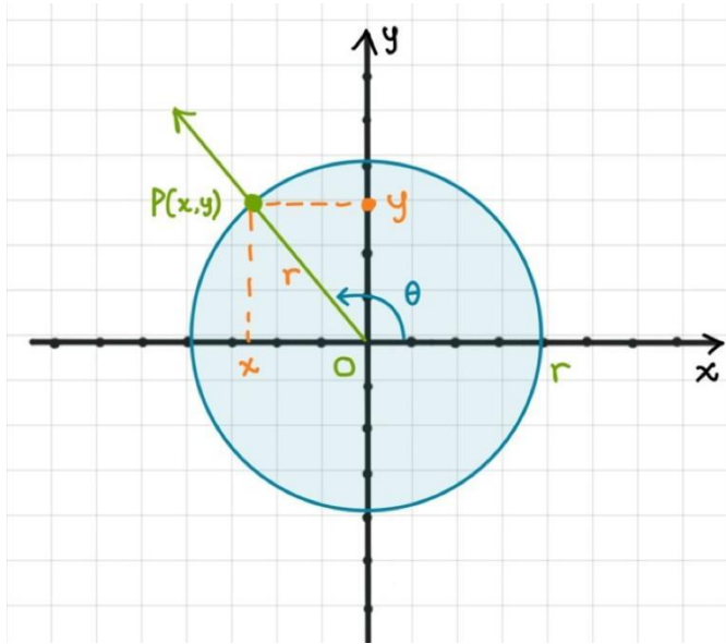
Gambar 5.5 Fungsi Trigonometri dari \theta dalam x,y dan r
