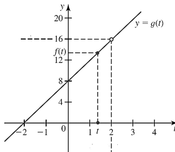
Gambar 6.1 Jika t Menghampiri 2, Maka g(t) Menghampiri 16.
