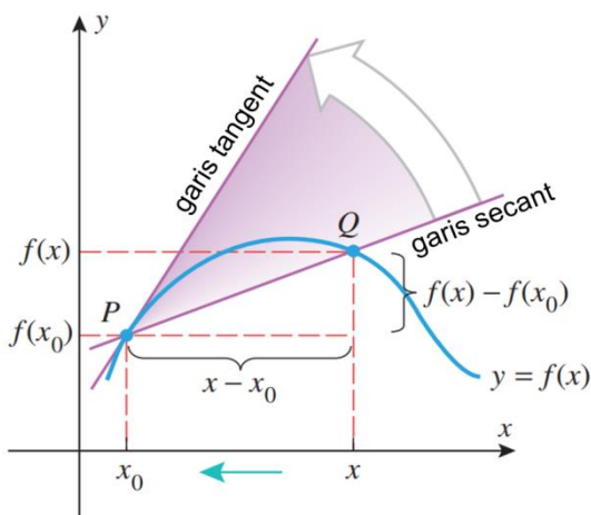
Gambar 9.2 Kemiringan Garis Singgung Kurva y = f(x) pada Titik P(x_0, f(x_0)) .
