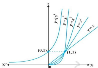
Gambar 5.1 Grafik Fungsi f(x) = x^n , n = 1, 2, 3, 4 dan f(x) = 10^x
