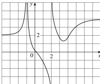
Gambar. 6.15 Grafik limit di tak hingga, dan asimptot dari f
