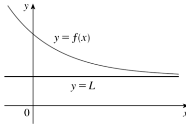
Gambar 6.14 Ilustrasi \lim_{n \rightarrow \infty} f(x) = L
