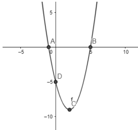
Gambar 4.2 Grafik Fungsi y = x^2 - 4x - 5 (Sumber: Geobegra)
