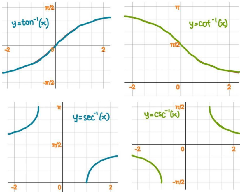
Gambar 5.11 Grafik Fungsi Siklometri Tan, Cot, Sec, dan Csc
