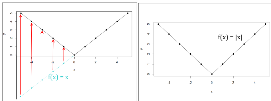
Gambar 3.1 Grafik f(x) = x yang dipantulkan ke y positif.
