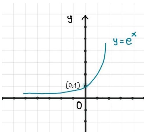
Gambar 5.3 Grafik Fungsi Eksponensial
