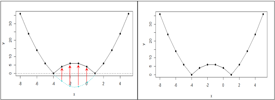
Gambar 3.3 Grafik |x^2 + 3x - 4| dengan Proses Refleksi Bayangan Negatifnya (Sumber: Penulis, 2023)
