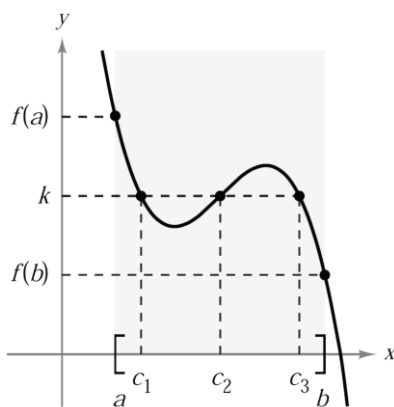
Gambar. 6.11 Fungsi f kontinu pada [a, b] . Terdapat tiga nilai c sehingga f(c) = k .
