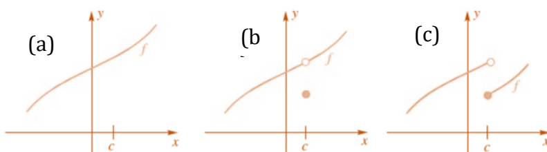
Gambar 8.1 Grafik Limit Suatu Fungsi \lim_{x \rightarrow c} f(x)
