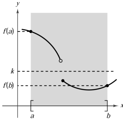
Gambar 6.12 Fungsi f tidak kontinu pada interval [a, b] .
