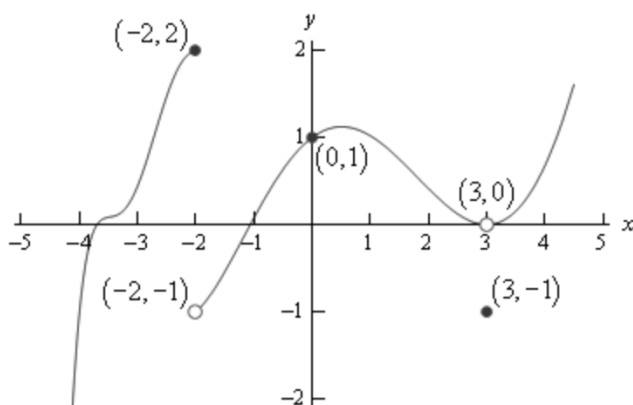
Gambar 8.2 Grafik Suatu Fungsi f(x)
