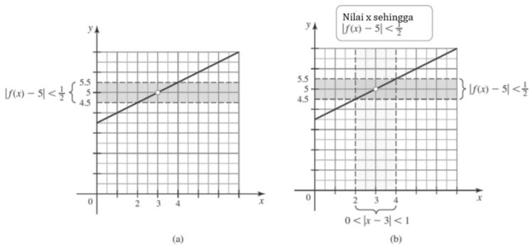
Gambar. 6.5 Grafik fungsi |f(x) - 5| < \frac{1}{2}
