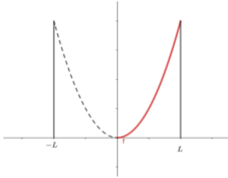
Gambar 4.8 Grafik Fungsi Genap
