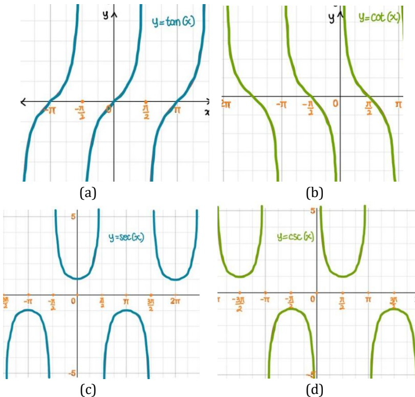
Gambar 5.9 Grafik Fungsi: (a) \tan(x) , (b) \cot(x) , (c) \sec(x) , (d) \csc(x)
