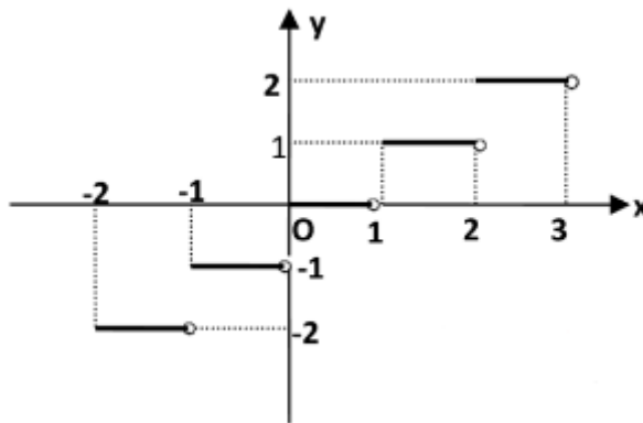
Gambar 7.1 fungsi bilangan bulat terbesar
