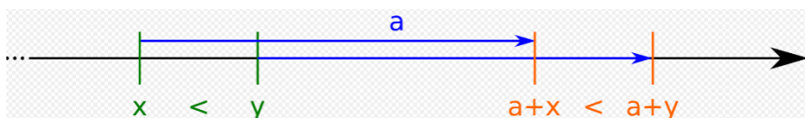
Gambar 1.2 Penambahan dan Pengurangan
