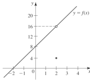
Gambar 6.3 Grafik fungsi f berimpit dengan fungsi g , kecuali pada titik x = 2 .
