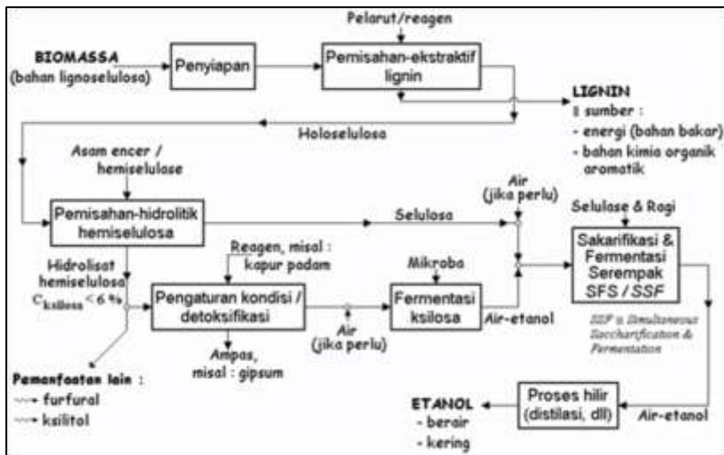
Gambar 10.9. Proses Pembuatan Bioethanol (sumber: https://th.bing.com )
