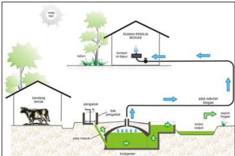
Gambar 10.6. Proses Pembuatan Biogas (sumber: https://2.bp.blogspot.com )
