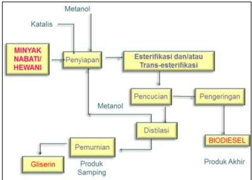
Gambar 10.8. Proses Pembuatan Biodiesel (sumber: https://ebtke.esdm.go.id )
